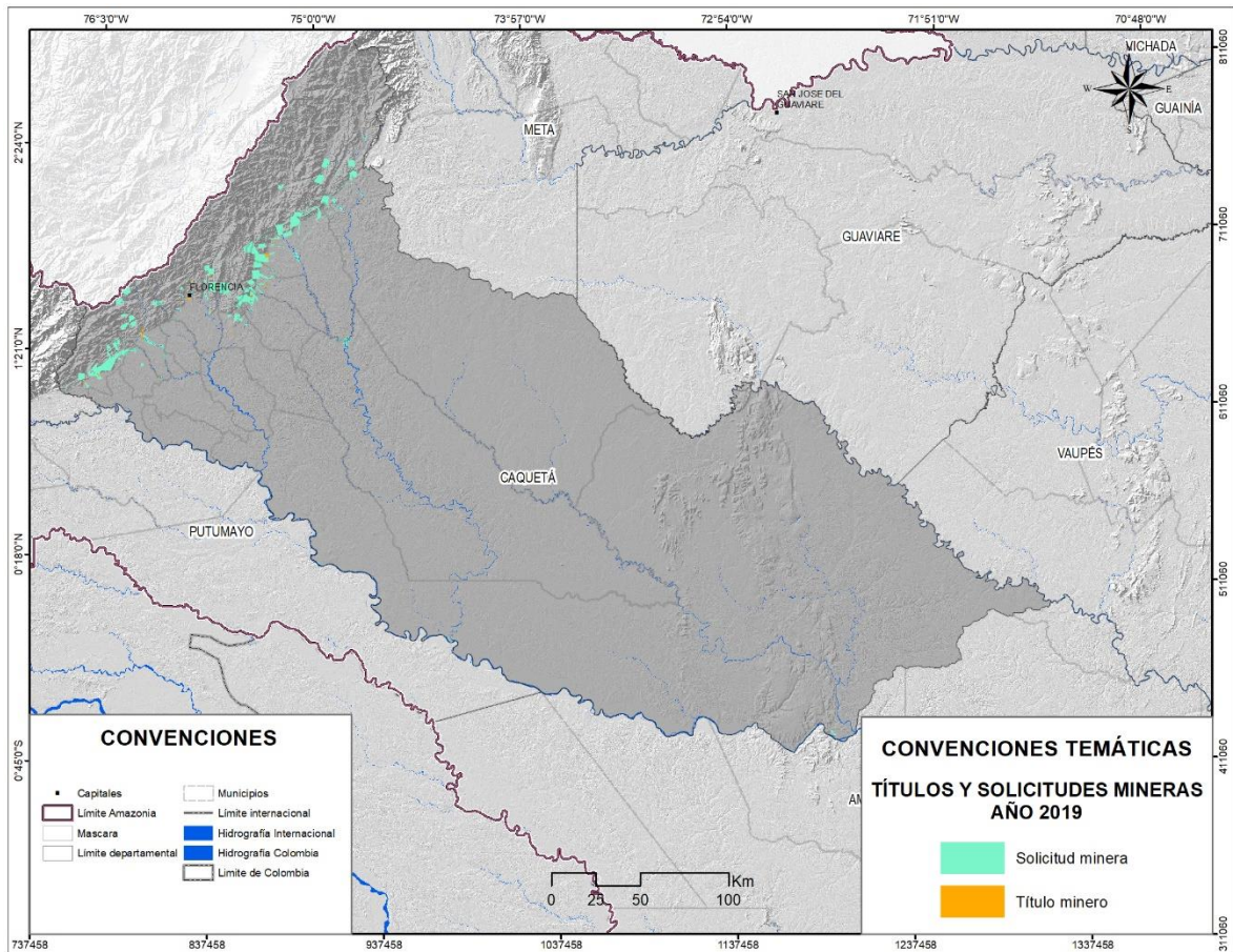
Figura 23. Títulos y solicitudes mineros 2019. Fuente: (ANM, 2019)
